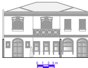
Elevation 02
